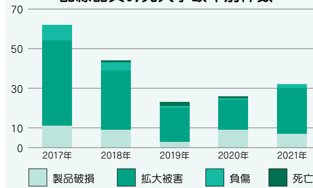
配線器具の発火事故年別件数
